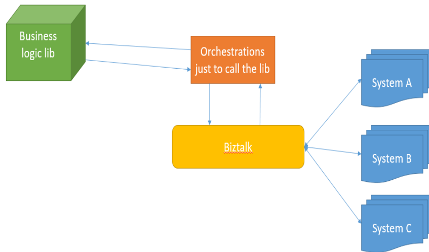
Рис. 1. Схема представлення бізнес логіки
