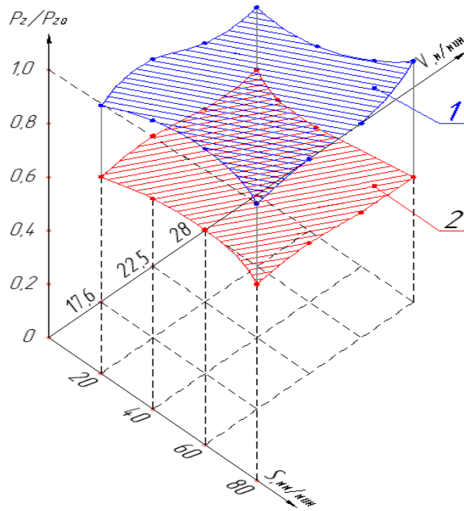
Рис.2 Вплив швидкості різання і подання на силу різання P_z при попутному фрезеруванні зразка з сталі 45 : 1 - "насухо"; 2 - з полімером (одношаровий поліетилен)
