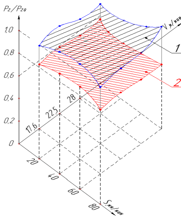
Рис.1. Вплив швидкості різання і подання на силу різання P_z при попутному фрезеруванні зразка з сірого чавуну СЧ20 : 1 - "насухо"; 2 - з полімером (одношаровий поліетилен)
