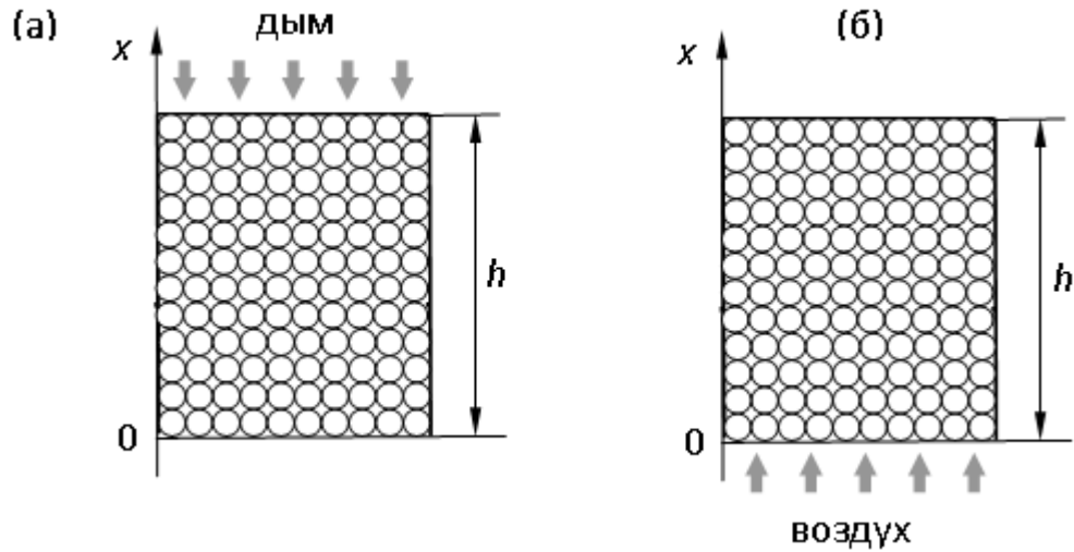
Рис. 1 – работы насадочного регенератора тепла Схема насадки регенератора в горячем (а) и холодном (б) периодах
