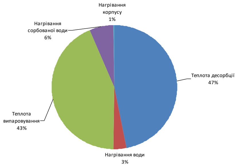
Рис.3 – Структура витрат теплоти на експлуатацію адсорбційного теплоакмулюючого пристрою відкритого типу при паровому зволоженні потоку повітря
