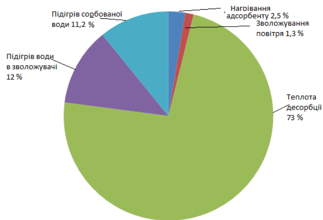
Рис.4 – Структура витрат на експлуатацію теплоакмулюючого пристрою відкритого типу при ультразвуковому зволоженні.
