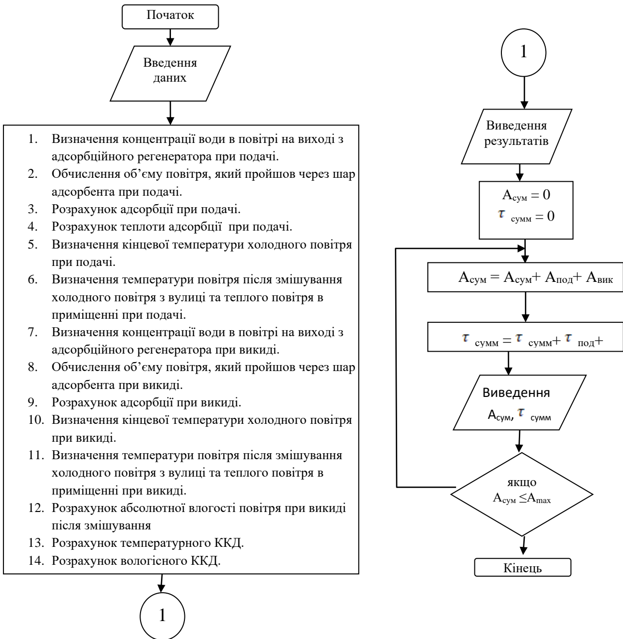
Рис. 2. Блок-схема алгоритму розрахунку адсорбційного регенератора
