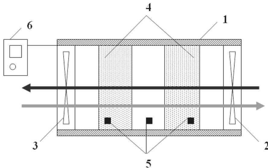
Рис. Конструкція регенератора тепла [3]
