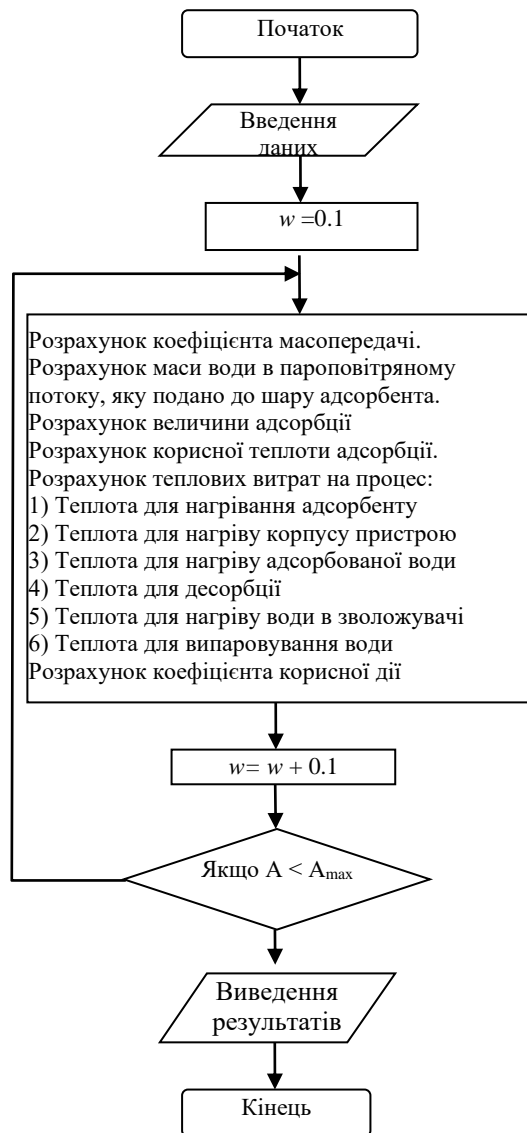
Рис. 2– Блок-схема алгоритму розрахунку коефіцієнту корисної дії адсорбційного теплового акумулятора
