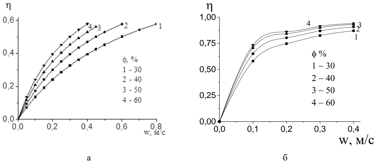
Рис. 5 – Залежність коефіцієнту корисної дії від швидкості пароповітряного потоку при відносній вологості 30 – 60 % та температурі 60°C. Товщина шару адсорбента 0,5 м.
