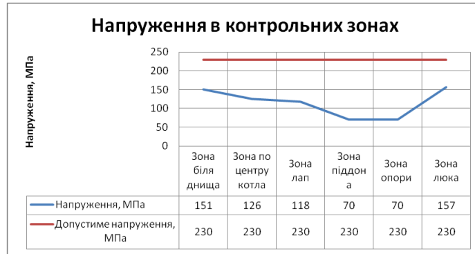
Рис. 7 – Графік напружень в контрольних точках під час ударних випробувань
