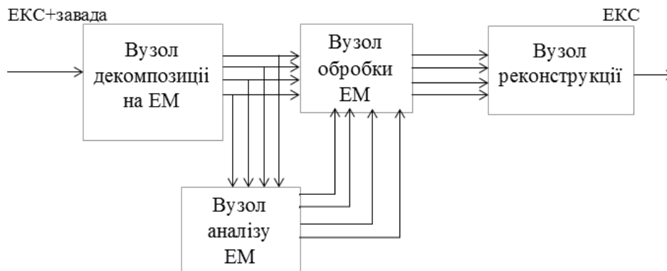
Рисунок 1. Структура реалізації процедури придушення завад в ЕКС на основі ДЕМ
